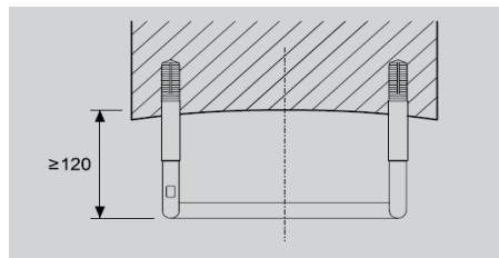
Obr. 5, 6 Umiestnenie stúpadiel
