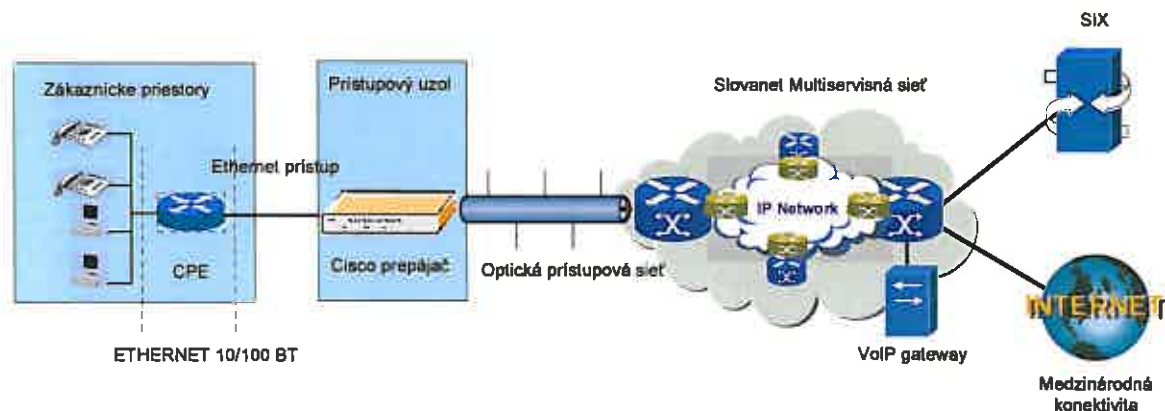
Obrázok: Schéma pripojenie do siete Slovanet
