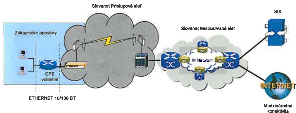
Obrázok: Schéma pripojenie do siete Slovanet
